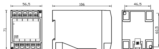
MPST-1, MPST-11, MPST-1-A e MPST-12-A
