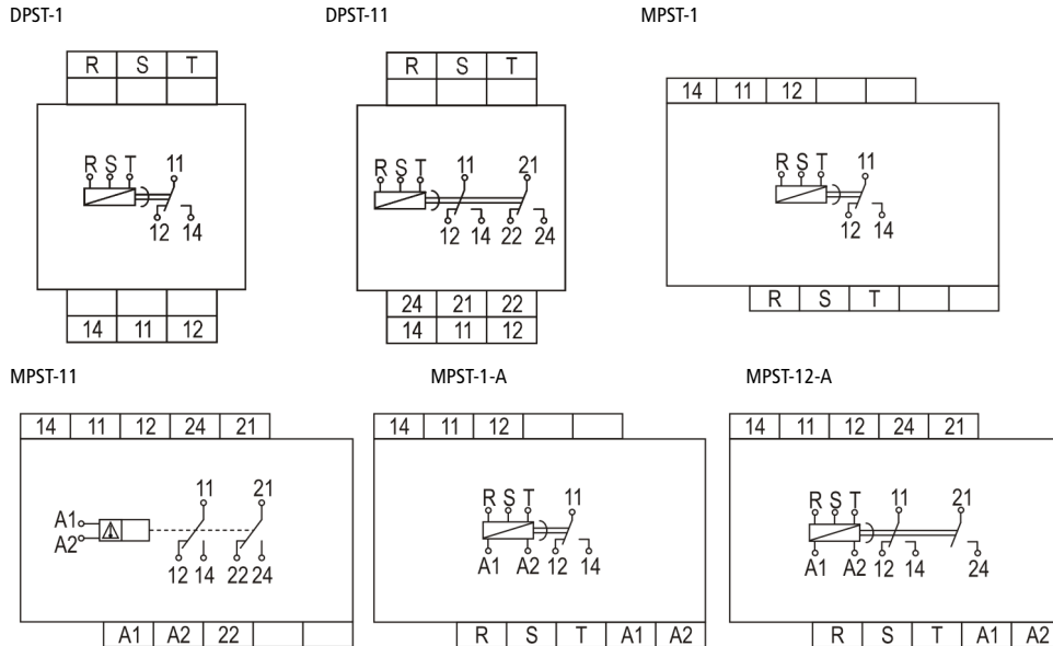
DPST-1 e DPST-11
