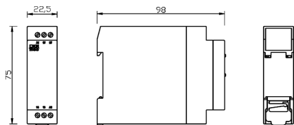
MPST-1, MPST-11, MPST-1-A e MPST-12-A
