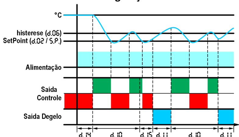
Gráfico 1 Funcionamento do modo refrigeração.
