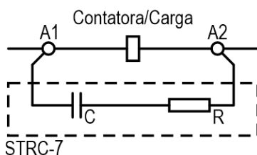
Figura 3 Esquema supressor de ruído elétrico e dimensões.
