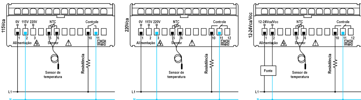
Esquema 2 Exemplos de ligação no Modo Aquecimento.
