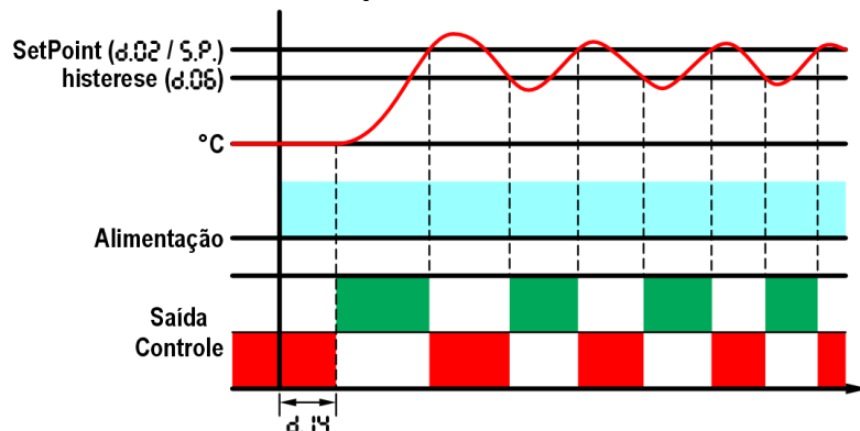
Gráfico 2 Funcionamento do modo aquecimento.
