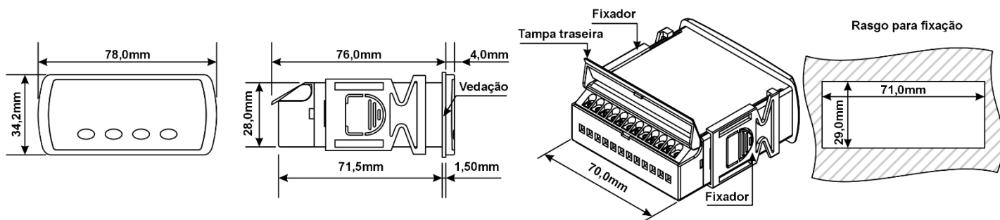
Figura 2 Dimensões.
